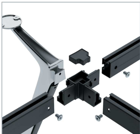
Schéma sestavení TR PS - prodlužovací spojky
