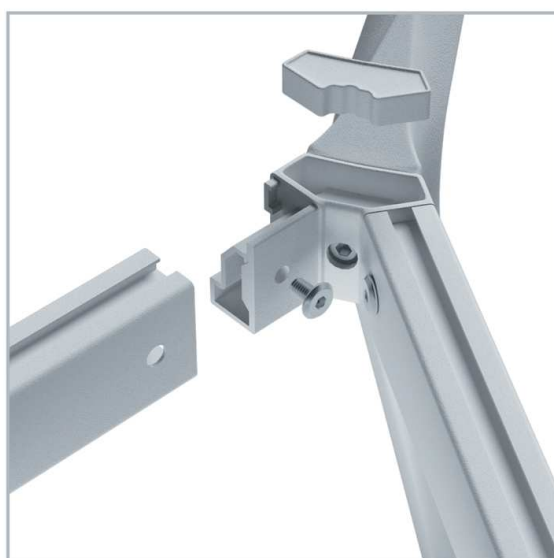
Schéma sestavení TR TS - trojúhelníkové spojky
